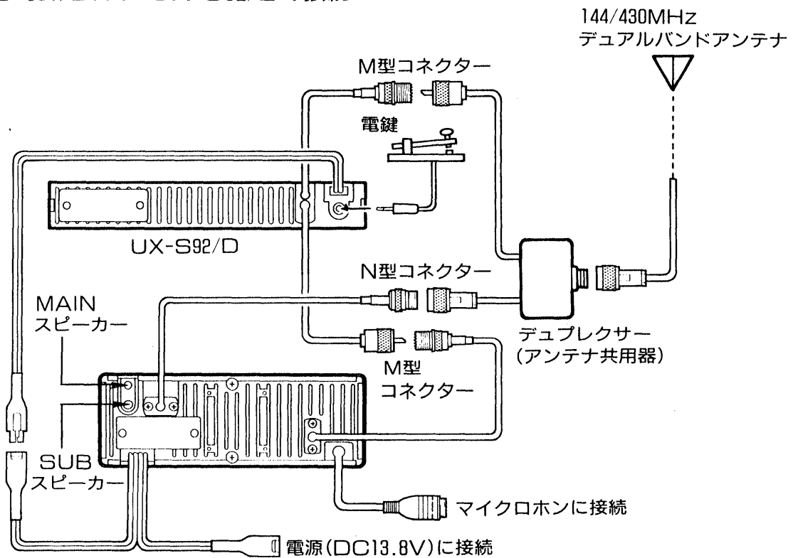
図26. IC-901/D/M+UX-S92/Dの接続
