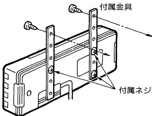
図6. リモートコントローラ部の取り付け
