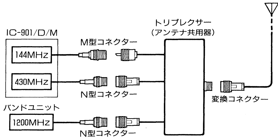
図20. トリプルバンドアンテナ接続例
