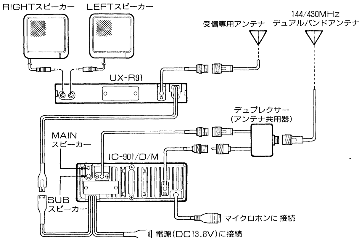
図24. IC-901/D/M+UX-R91の接続
